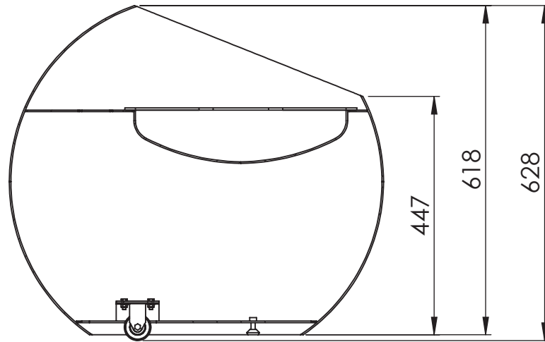
COUPE A-A
